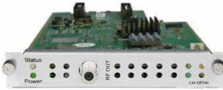
CM2-OFDM-R01: OFDM Modulation Module
