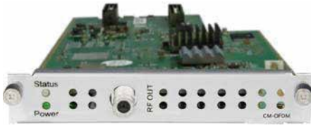
CM2-OFDM-R01: OFDM Modulation Module
